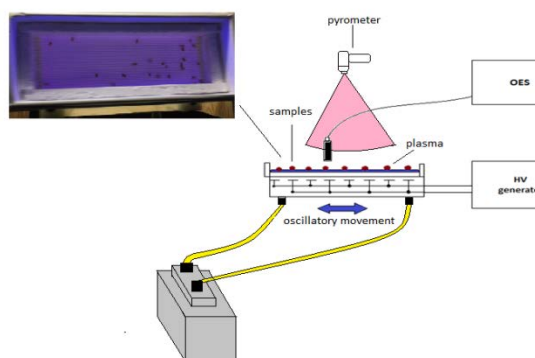
Рисунок 1 - Общий вид экспериментальной установки
